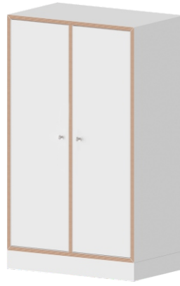
Schrank, 3 Ordnerhöhen, 2 Türen mit Schloss Einlegeböden: 4 B/H/T: 70,1 × 110,5 × 42,6 cm
